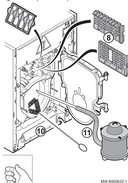
Fig.74 Limpeza do corpo de caldeira
