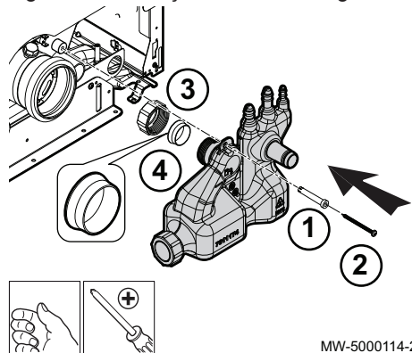
Fig.14 Colocação do sifão no lugar
