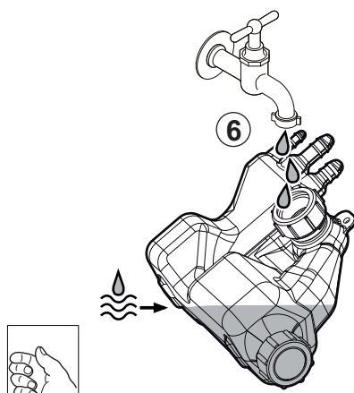
Fig.37 Processo de enchimento
