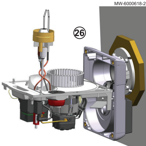
Fig.79 Limpeza do ventilador
