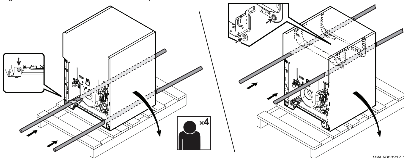
Fig.12 Manuseamento com barras de transporte
