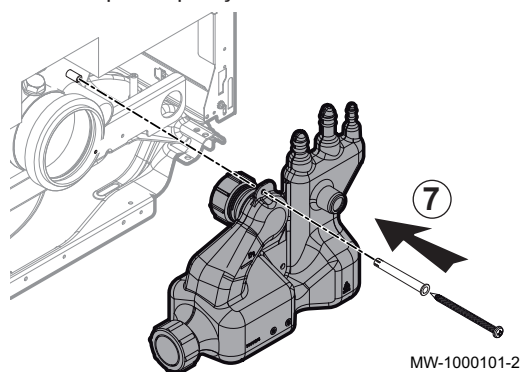
Fig.38 Voltar a colocar o sifão na sua respectiva posição
