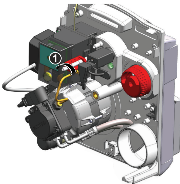
Fig.48 Regulação da fenda de recirculação
