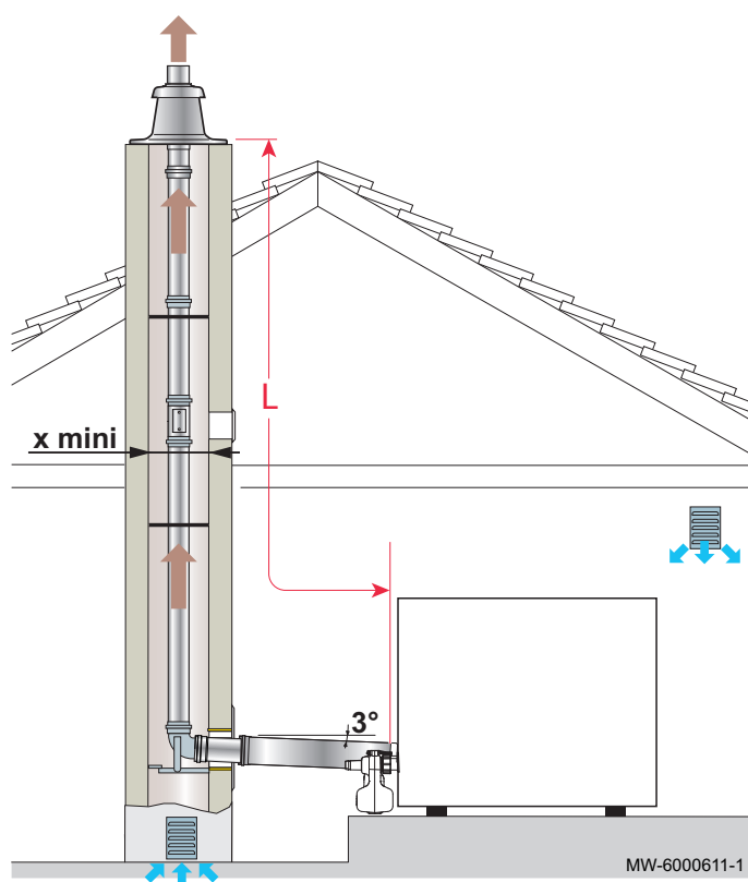
Fig.16 Ligação rígida tipo B 23P - Conduitas de evacuação de fumos (ar de combustão tomado da sala da caldeira)
