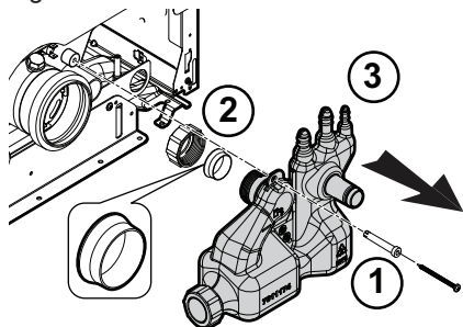
Fig.36 Remover o sifão
