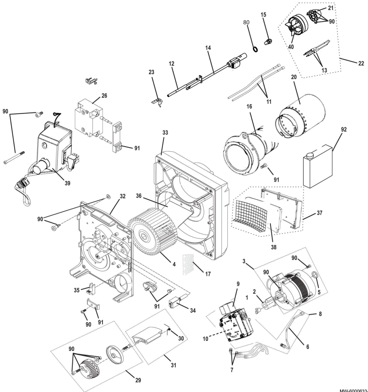
Fig.92 Queimador
