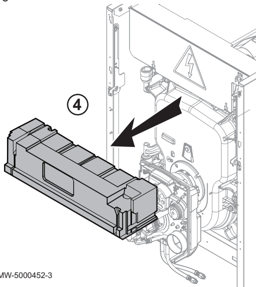
Fig.72 Remover o queimador
