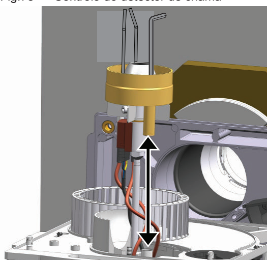
Fig.78 Controlo do detetor de chama
