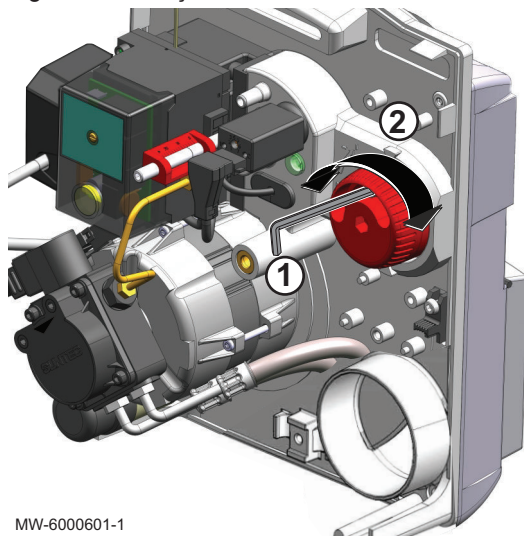
Fig.47 Definição da entrada de ar
