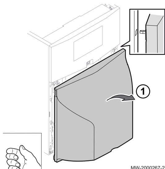
Fig.69 Remover o painel dianteiro superior
