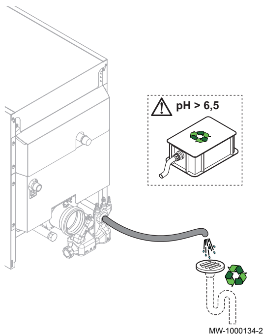
Fig.15 Ligação da conduta de evacuação dos condensados
