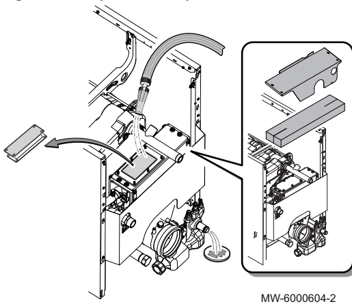
Fig.75 Limpeza do corpo do condensador
