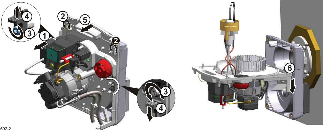
Fig.76 Colocação do queimador na respetiva posição
