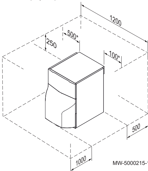
Fig.8 Espaço a prever
