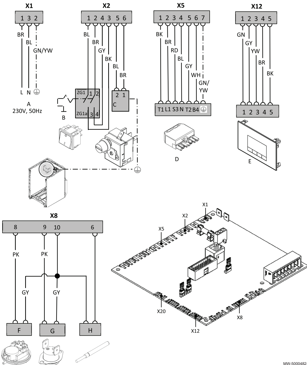
Fig.3 Esquema eléctrico
