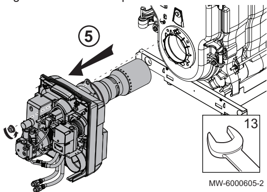
Fig.72 Remover o queimador
