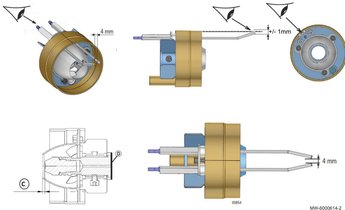
Fig.49 Espaçamento nos elétrodos de ignição
