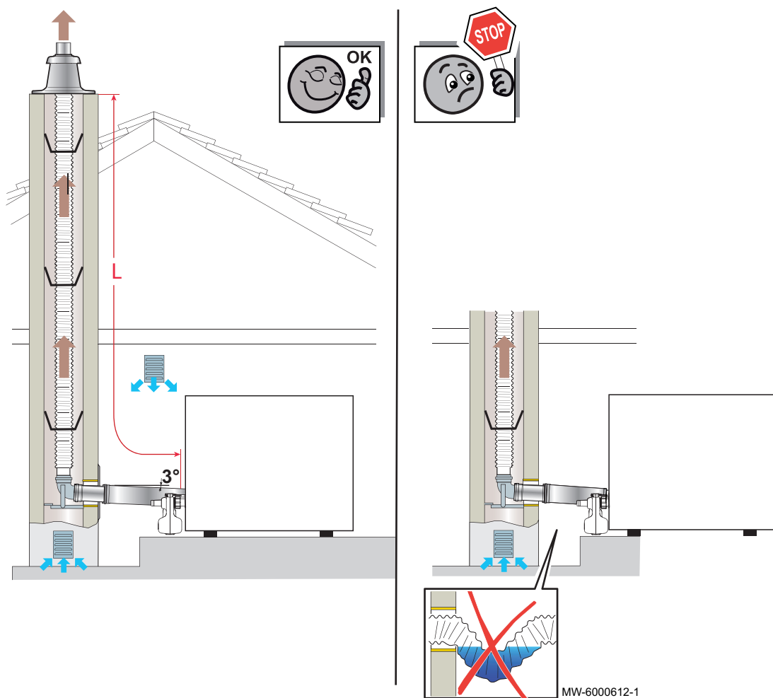
Fig.17 Ligação flexível tipo B 23P - Condutas de evacuação de fumos (ar de combustão tomado da sala da caldeira)
