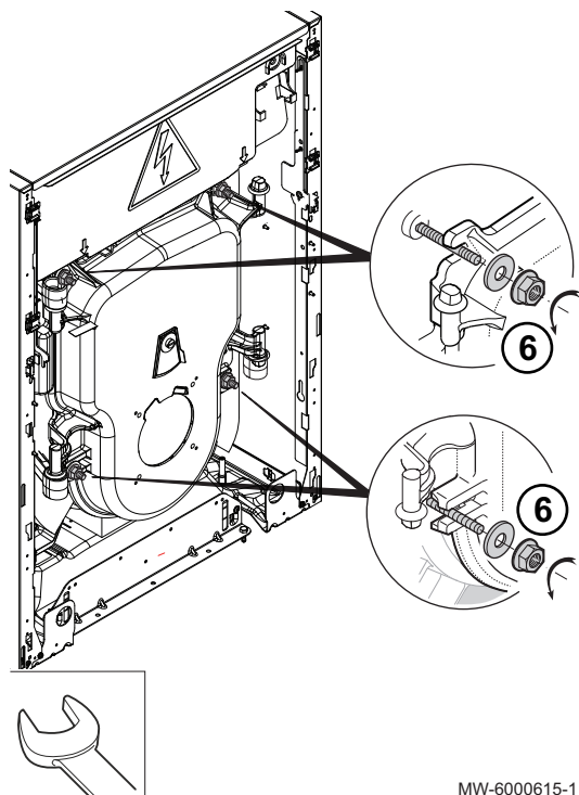
Fig.74 Limpeza do corpo de caldeira
